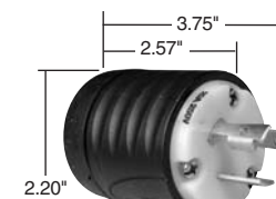
20A Plug
