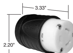
30A Connector
