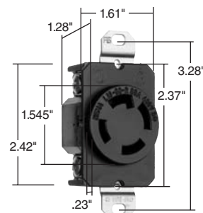
30A Receptacle
