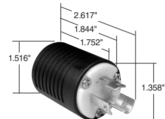
15A Plug
