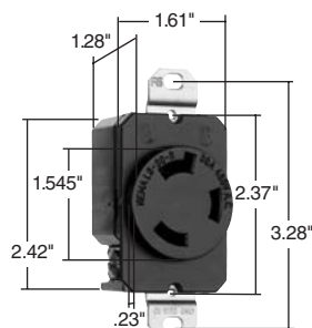
30A Receptacle
