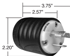
20 & 30A Plug
