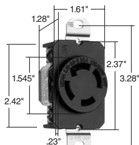
30A Receptacle
