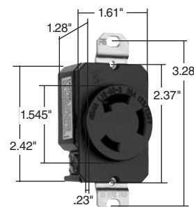
30A Receptacle
